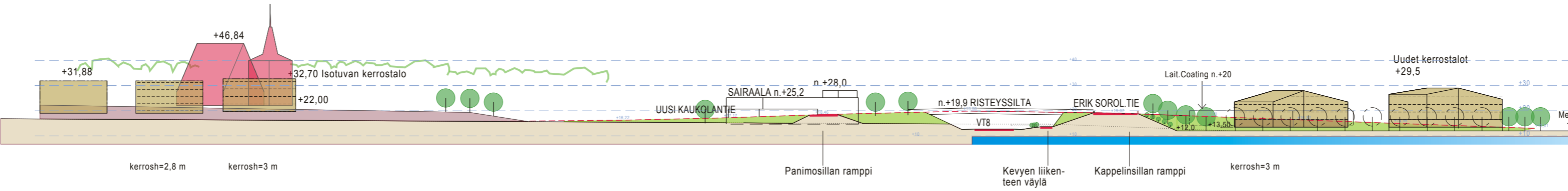
MAASTOLEIKKAUS KAUKOLANTIEN - ERIK SOROLAISEN TIEN SUUNTAISESTI, VALTATIE RISTEYSSILTA
